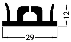
AC135/A – GUIDA ZIP mm.29 PER AC135 L/ mm.6000 PACCO / 1 BARRA
