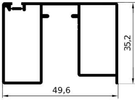
GA1594 – gr/ml 618 MIN KG.500
